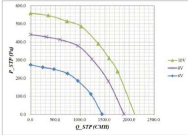
流量-压力/P-Q
