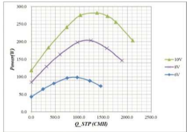
流量-功率/Q-W
